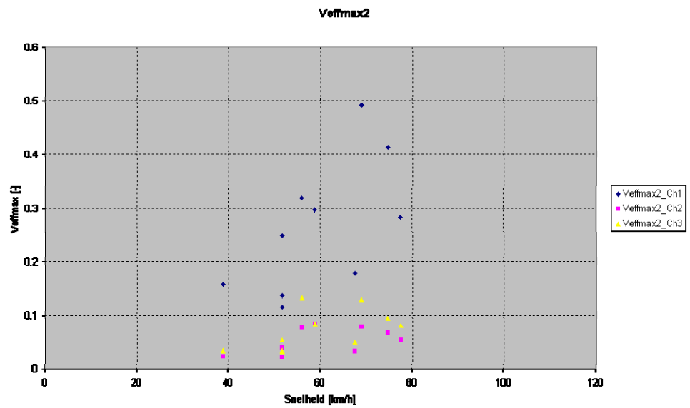
Figuur 24: Trillingsniveau tegen treinsnelheid bij referentieband 2 (voor treinpassages van Captrein België).
